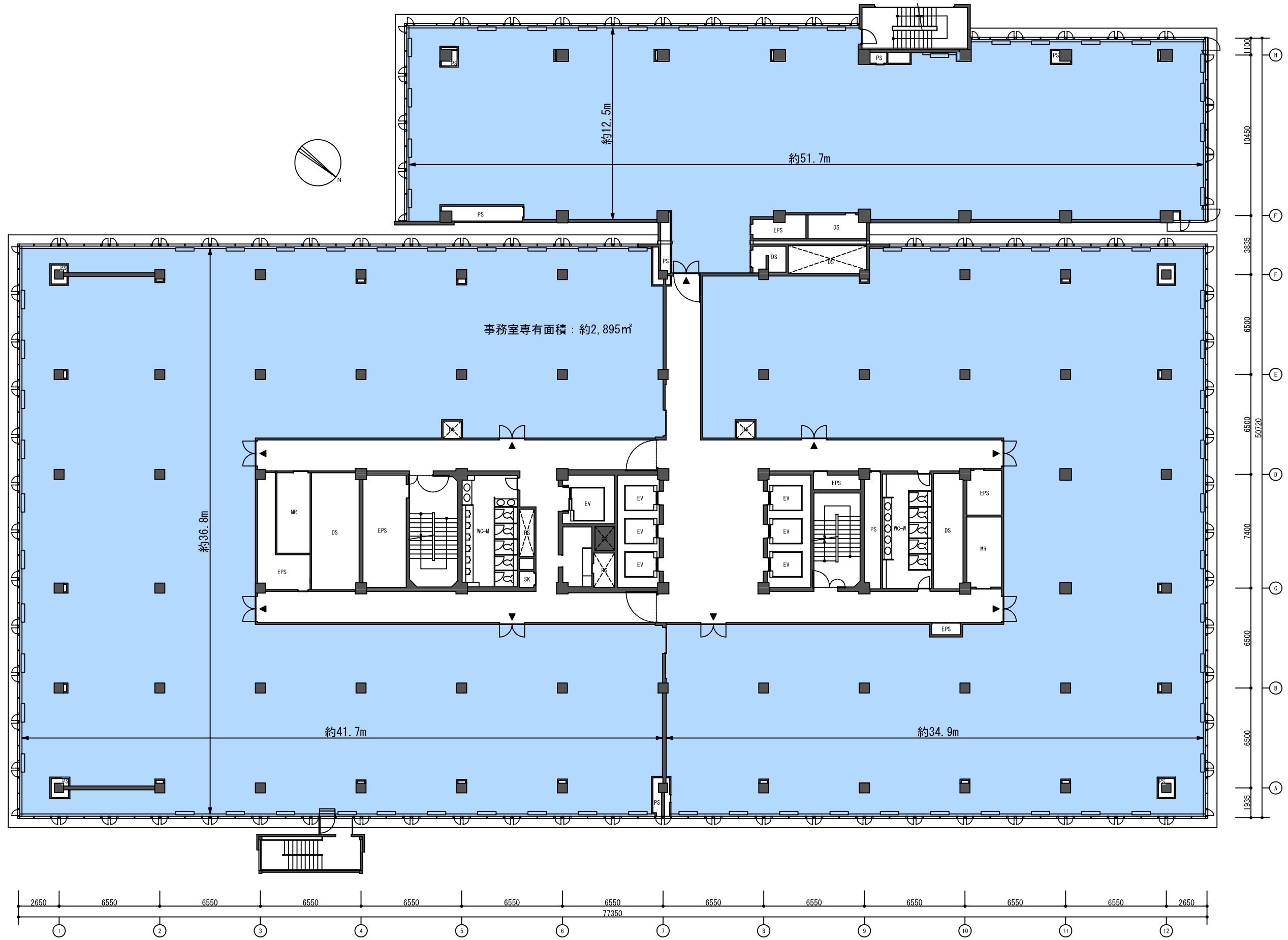
第一田町ビル 基準階平面図
