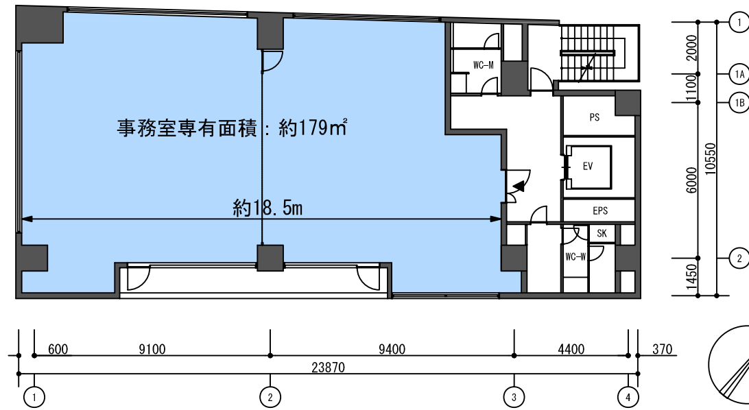
三田ステーションビルアミタ 基準階平面図
